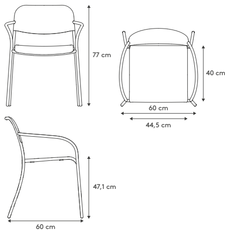
Product Dimensions 62172+62175+62178+62181 | Produktabmessungen Armlehnenstuhl 62172+62175+62178+62181
