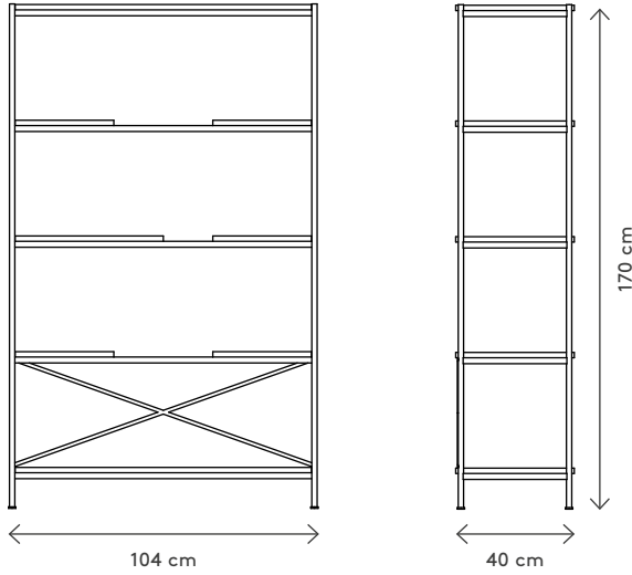
Product Dimensions 67315 + 67316 | Produktabmessungen 67315 + 67316
